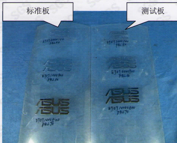
盐雾试验后
